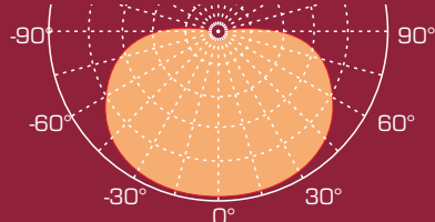
Light Distribution Curve Светлоразпределителна крива
